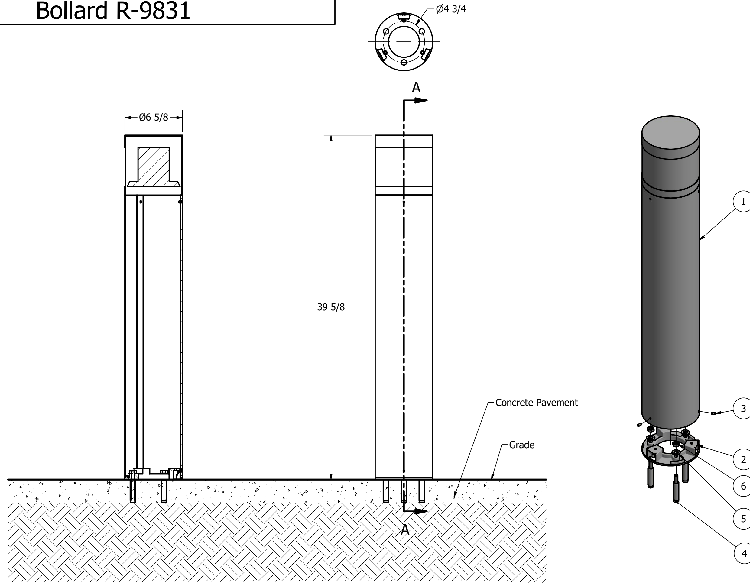
SECTION A-A
