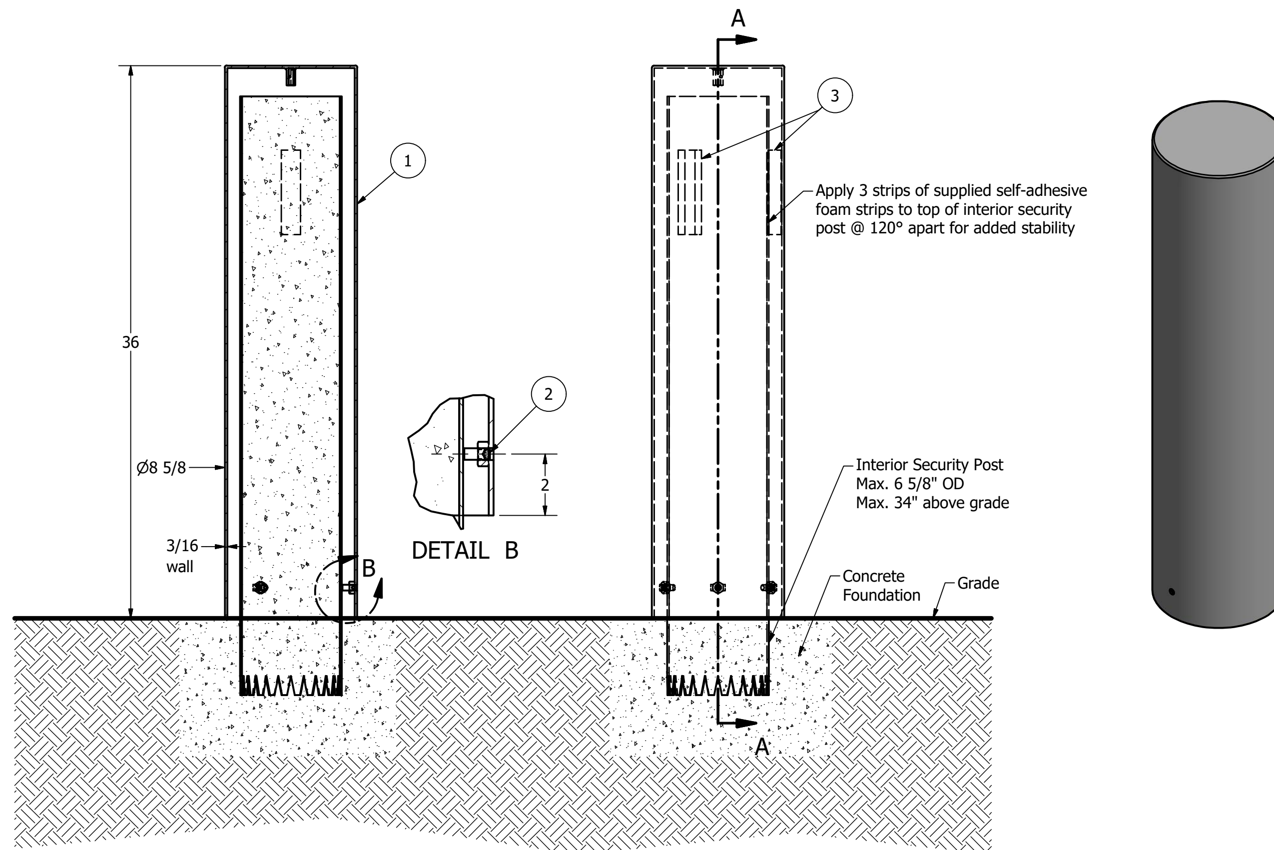
SECTION A-A
