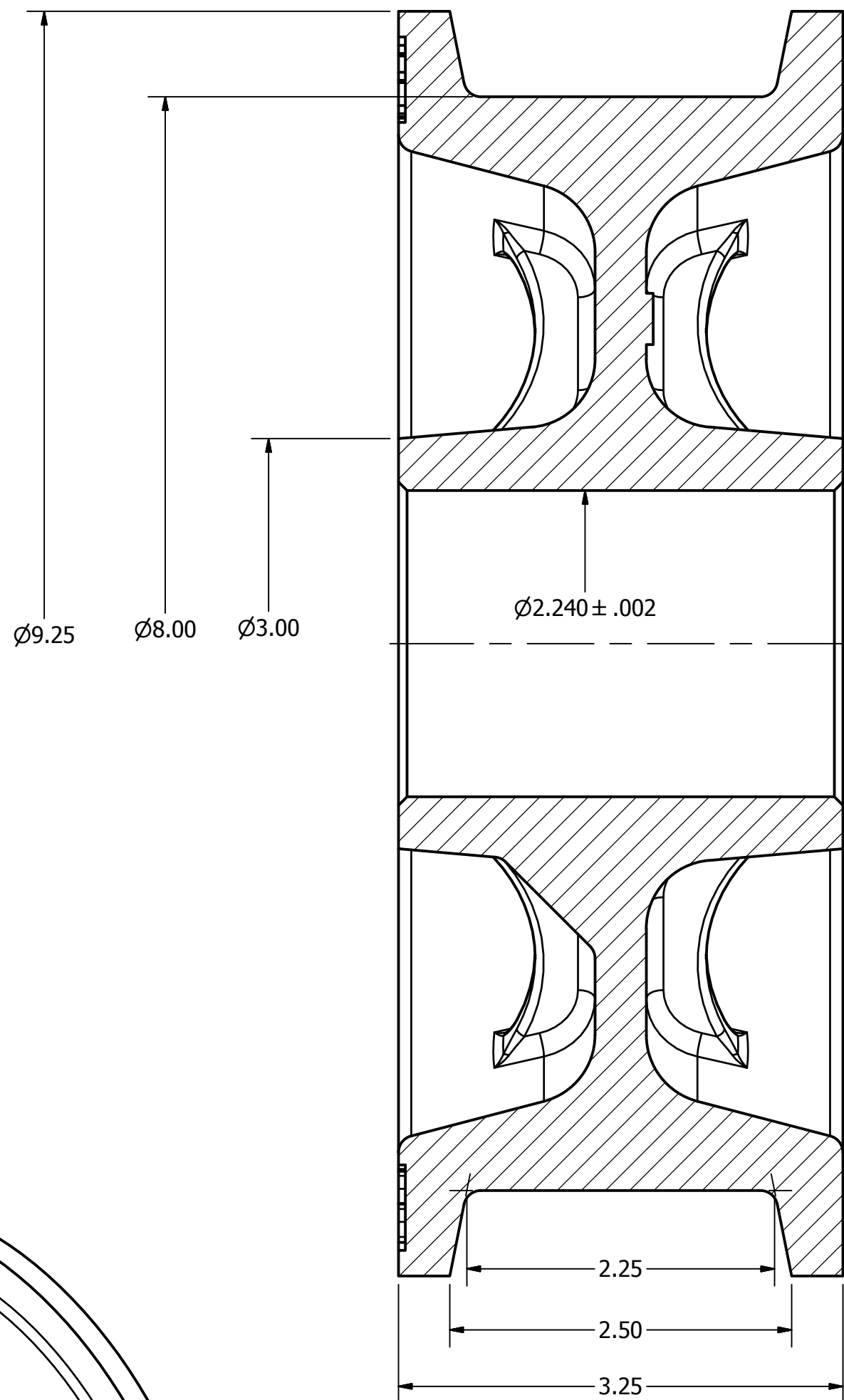
SECTION A-A
