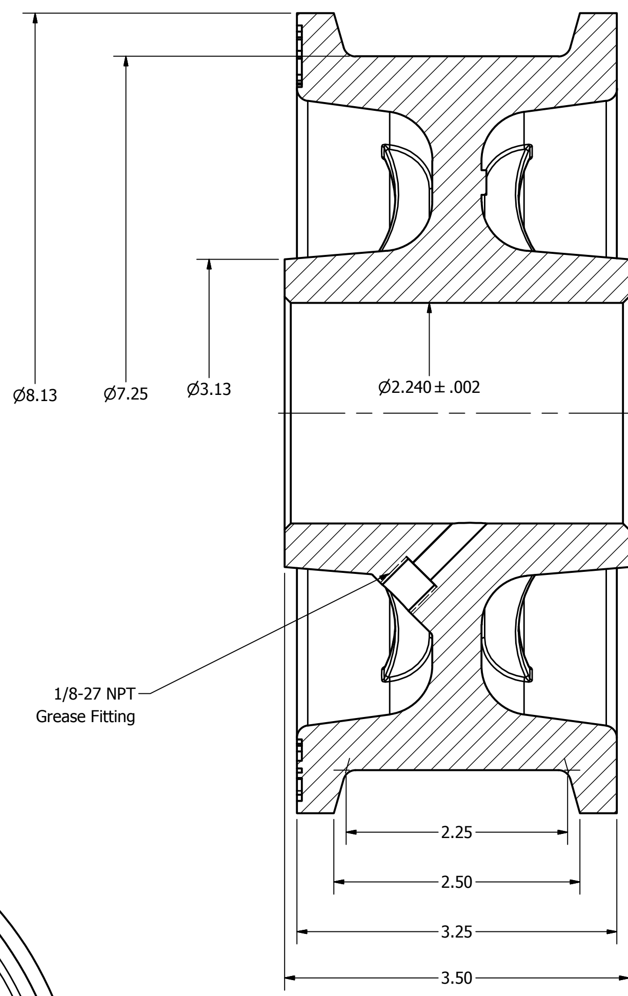
SECTION A-A
